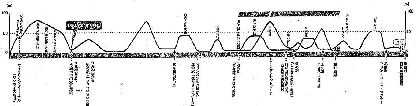
(瀬戸内海横断自転車道 高低表)
